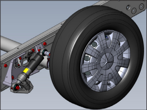
Luftfederung: Air Premium X2 hinten – Heck anheben/absenken (ca. +/- 50 mm gegenüber der Fahrposition). Air Premium X4 vorne/hinten – vorne/hinten anheben/absenken (wie oben). Nivellierfunktion für ebenen Stand. (nicht für Light-Ausführung, TRAQ x750 und X4 nicht für TRAQ i830)
