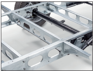
Chassis-Paket 4.250 kg Chassis-Paket 4.400 kg (in Verbindung mit 180 PS-Motor)
