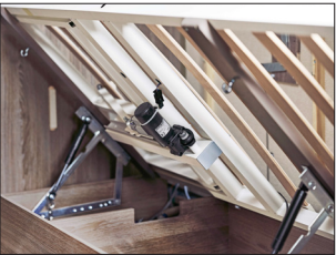
Sähköinen pääty sängyssä (vakiona kaikissa LQB-malleissa). Lisävarusteena takatallin korkeus pienenee 10 cm.
