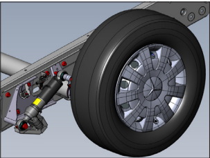
Ilmajousitus: Air Premium X2 taakse – nosta/laske takapäätä (n. +/- 50 mm ajoasennosta) Air Premium X4 eteen/taakse – nosta/laske edestä/takaa (kuten yllä). Tasausjärjestelmä vaaka-asentoon (ei Light-mallissa, ei TRAQ x750 ja X4 ei TRAQ i830 -malliin)
