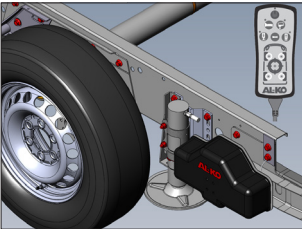
AL-KO HY4 -hydrauliset tukijalat
