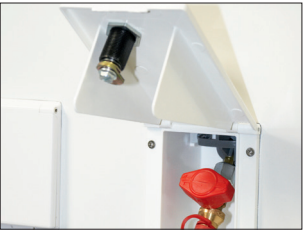
Prise de gaz extérieure (GPL)
