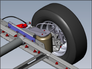
AL-KO Comfort Drive ACD Actieve schokdempers die de damping bliksemsnel aanpassen aan de rij situatie. Meer comfort, meer stabiliteit en wegligging en een preciezere besturing. (c720, x750, i780, x810 Heavy-uitvoering)
