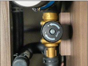
AGS II Pro verwarmingssysteem (inbegrepen in Prime-Comfort, standaard Imperial)
