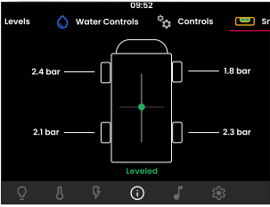
KABE Smart Level med tre praktiska funktioner håller koll på gasolen**, däcktrycket och fordonets lutning (standard Imperial). KABE Smart Level styrs via KABE Smart D 2.0 panelen.
