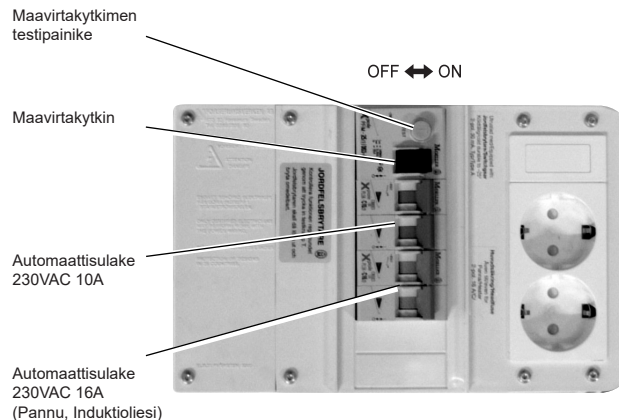
Sähkökotelon takaosa
