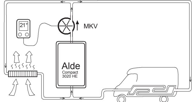
Kuva 1: Kaaviokuva asunto-osan lämmitysjärjestelmästä.
