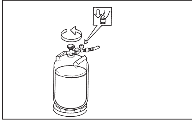
Letkunrikkoverttiili on asennettu kaasuletkuun.
